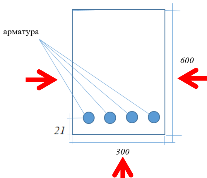
Рисунок 2. Переріз залізобетонної балки.
