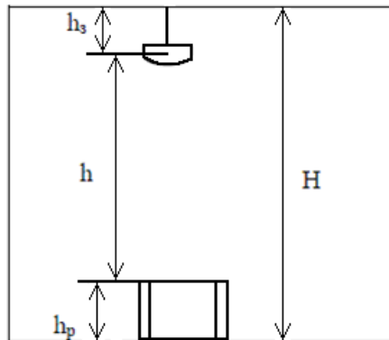
Рисунок 1.1 – Схема розміщення світильників над робочою поверхнею ( H – висота приміщення, м; h_3 – висота звисання світильника від стелі, м; h – висота підвісу світильника над робочою поверхнею, м; h_p – висота робочої поверхні, м.)
